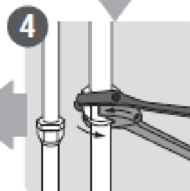
Conecte las tuberías del refrigerante
