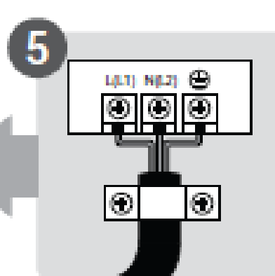
Conecte los cables
