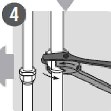
4 Conecte las tuberías del refrigerante
