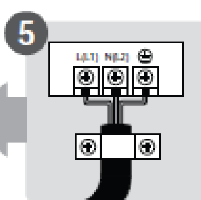
5 Conecte los cables
