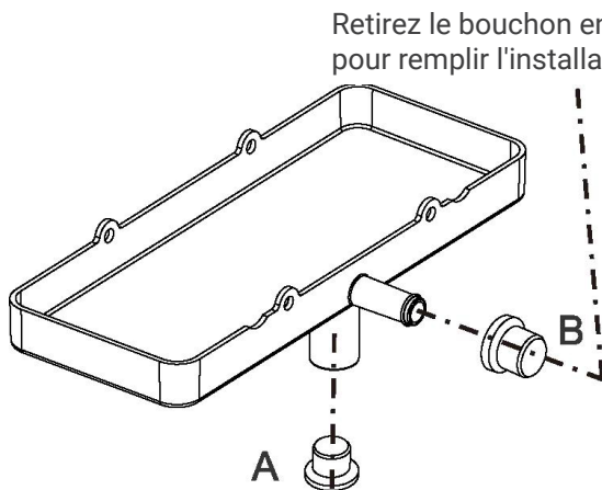
Retirez le bouchon en caoutchouc A pour remplir l'installation verticale
