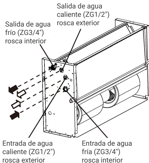
Sistema 4 tubos
