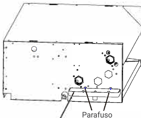
Bandeja de drenagem auxiliar para instalação horizontal.
