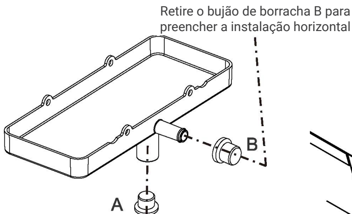
Retire o bujão de borracha A para preencher a instalação vertical
