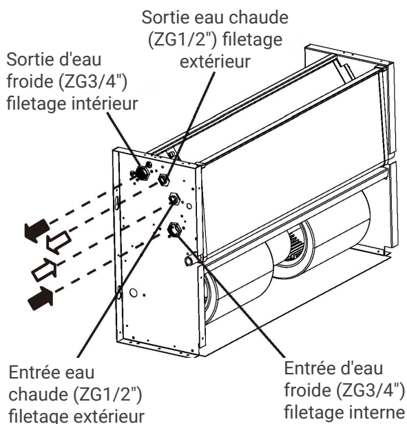
Système à 4 tubes
