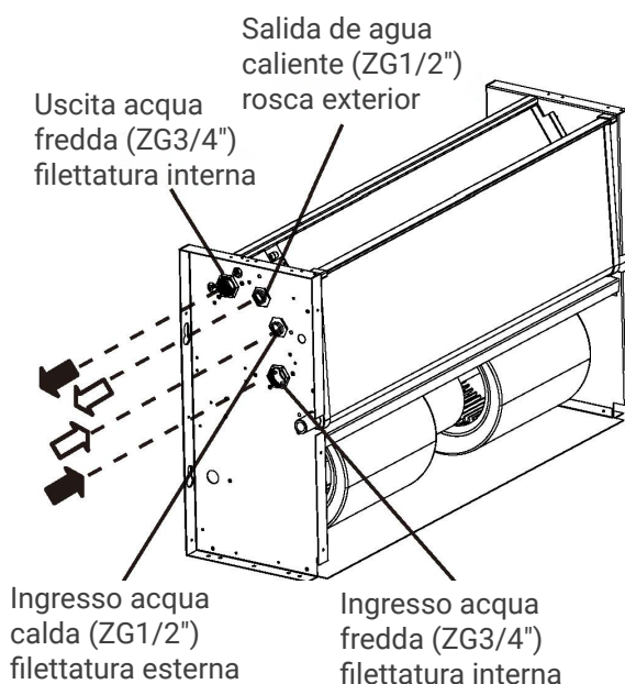
Sistema a 4 tubi
