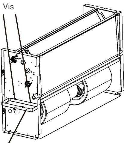
Bac de récupération auxiliaire pour installation verticale.
