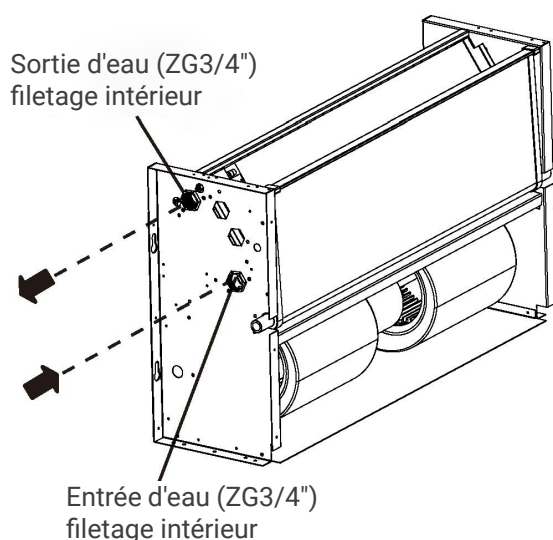
Système à 2 tubes
