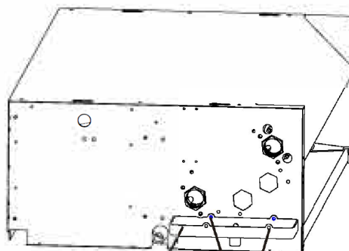
Bandeja de drenaje auxiliar para la instalación horizontal.
