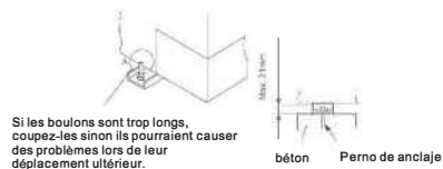
Fig. 2 Installation de boulons d'ancrage
