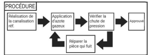
Procédure de scellement
