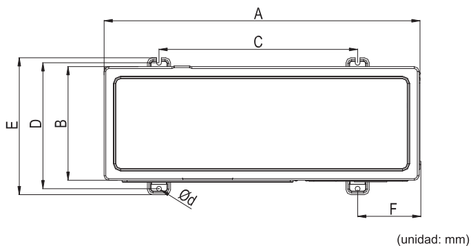
Fig. 2 Instalación de los pernos de anclaje
