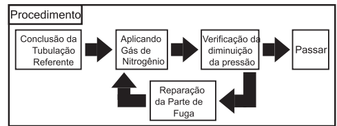
Procedimento de estanquidade
