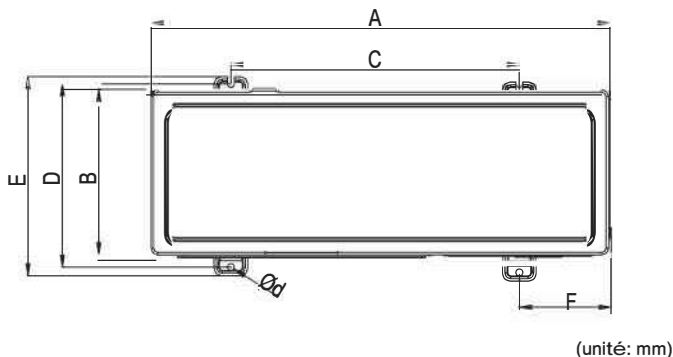
Fig. 2 Installation de boulons d'ancrage
