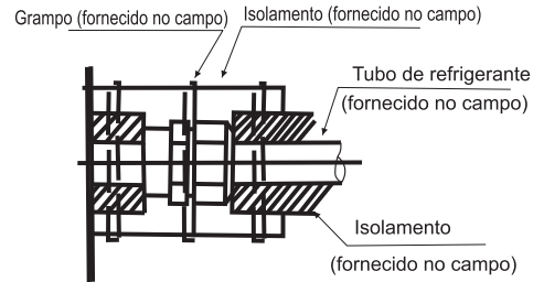
Procedimento de isolamento de tubulações
