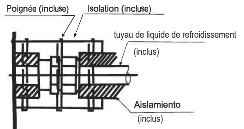
Procédure d'isolation des tuyaux
